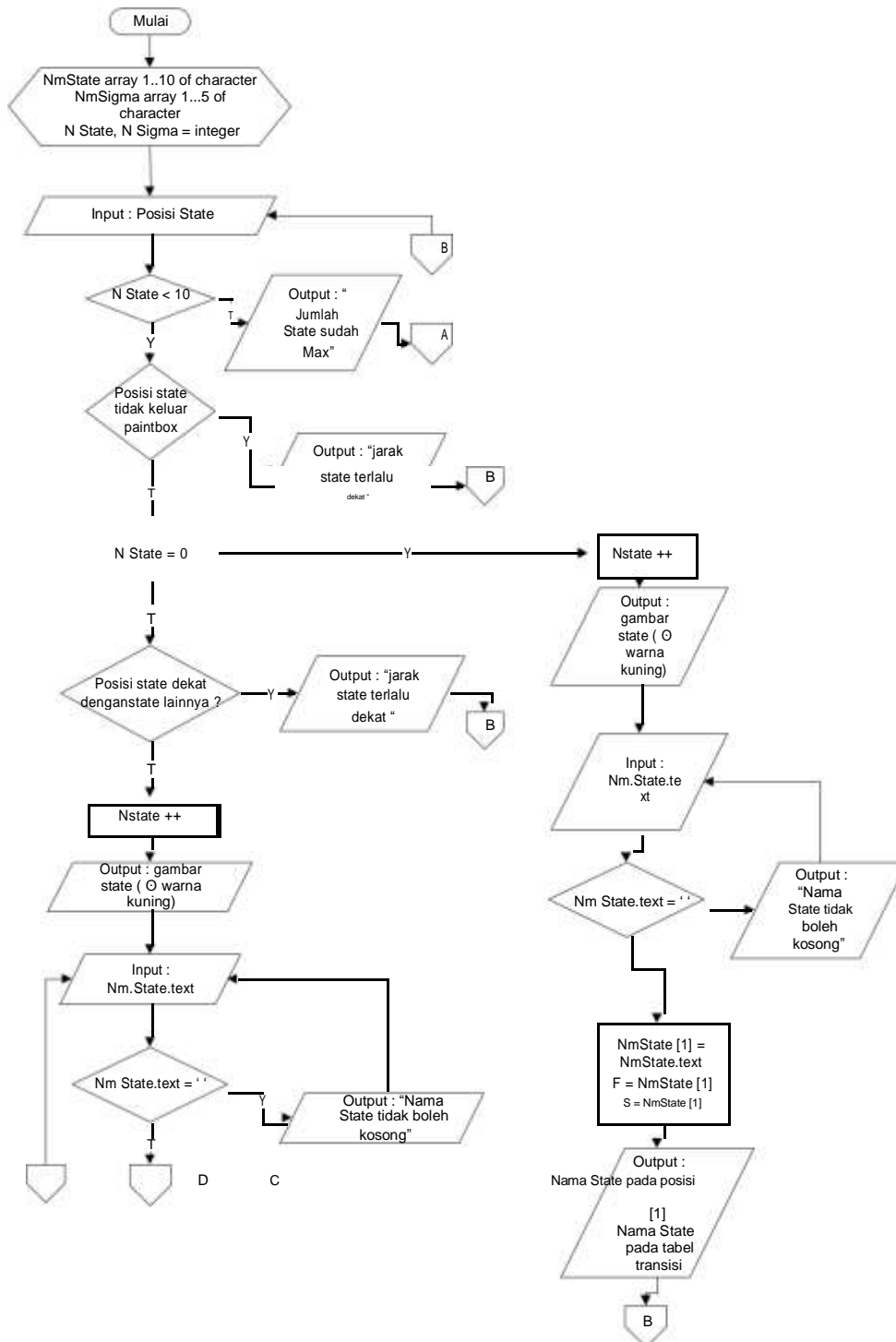
Gambar 4. Flowchart Algoritma Aplikasi FSA (versi.1)
