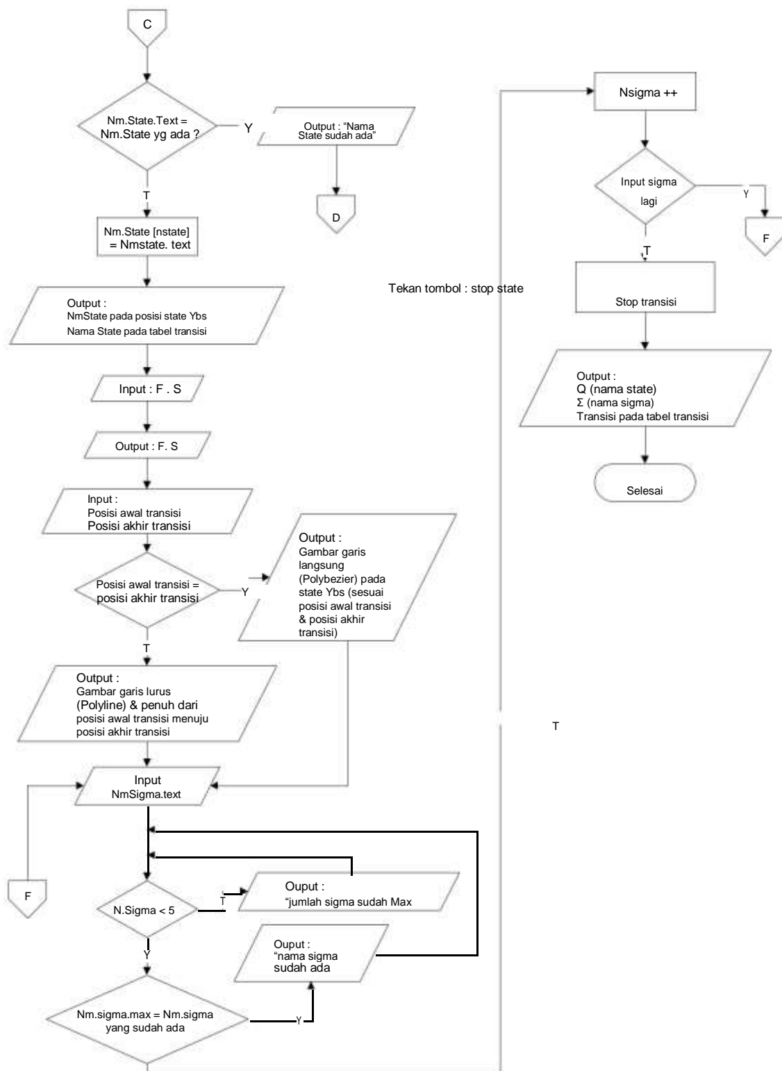
Gambar 5. Flowchart Algoritma Aplikasi FSA (versi.1) (Lanjutan)
