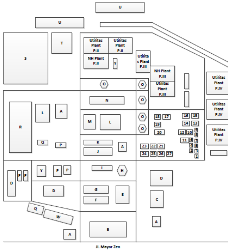
Gambar I.2 Layouts kompleks PT Pusri Palembang
