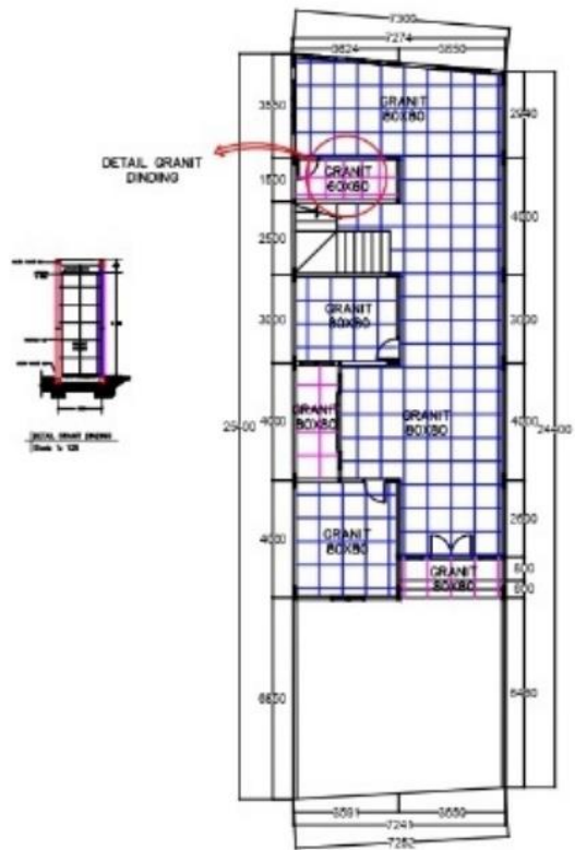
DENAH POLA LANTAI LT. 1 SKALA 1:200
